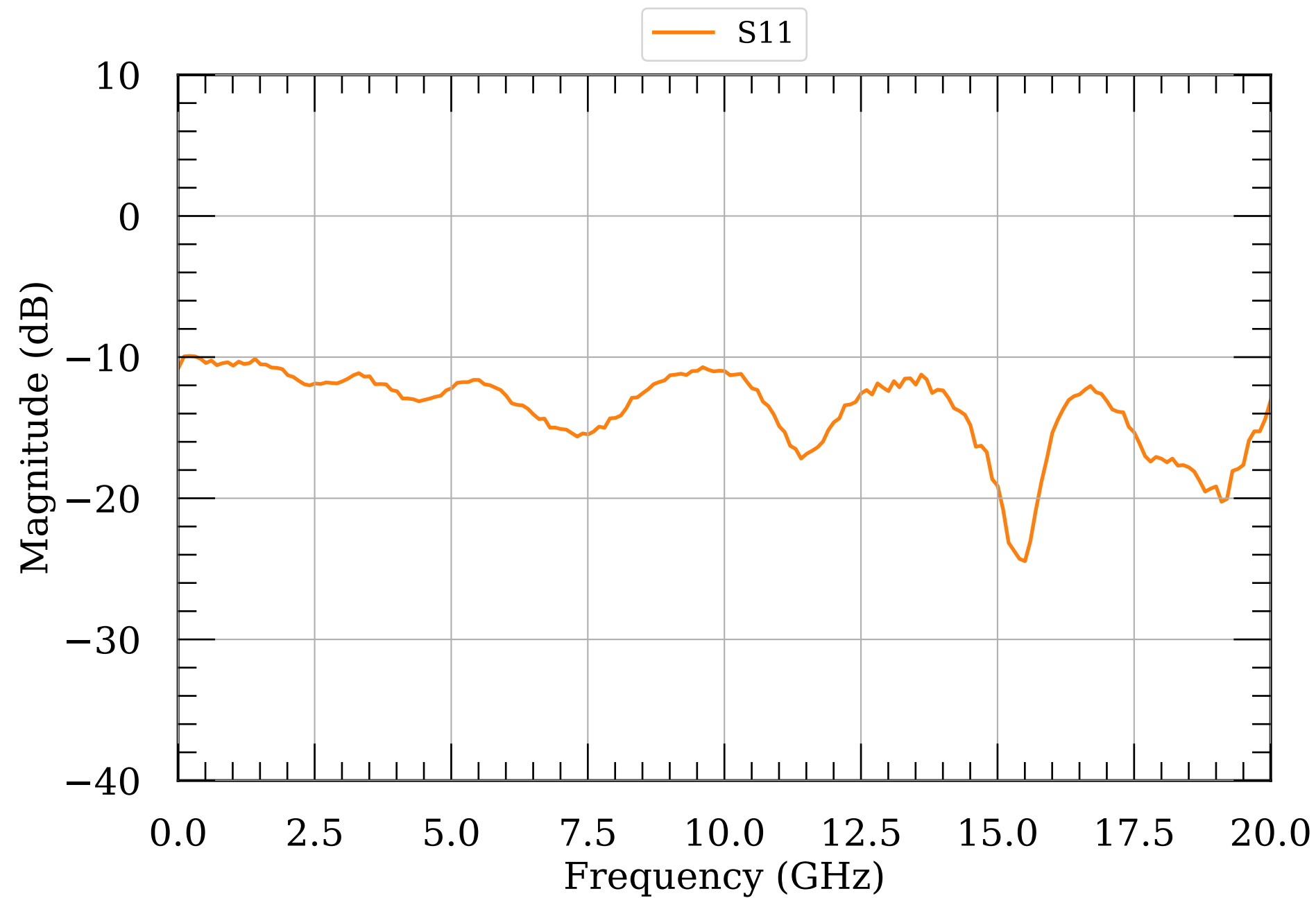
LNA S-params module090
